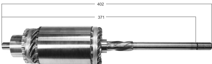
321111 REFORMA AN 115 12V. EJE SUPER LARGO GIRO IZQ. (ARRANQUE 301469I)
