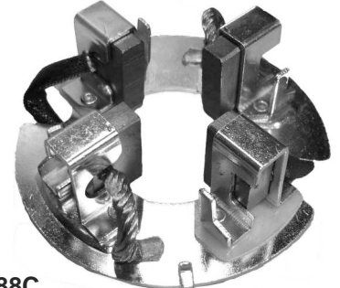
P2288C ARR. INDIEL, M. BENZ MOTOR CUMMINS - MWM - 8 x 25 x 16
