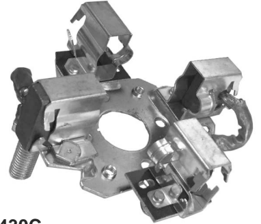
P2430C PORTAESCOBILLAS ARRANQUE TIPO BOSCH
