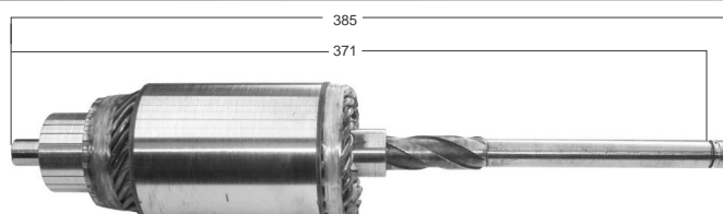
321110 REFORMA SOMECA AN 115 24V. EJE SUPER LARGO (ARRANQUE 301469/24)
