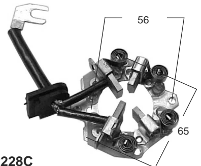
P2228C ARR. HITACHI, CORSA - ASTRA DIESEL 4.5 x 14 x 15.5 (352 58 566)
