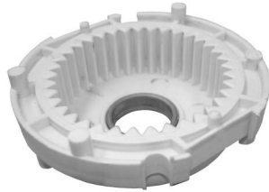
P1321 MOTORCRAFT, TRANSIT BUJE ALTURA 6mm-eje ø17,5 Z37
