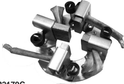
P2179C PORTAESCOBILLAS ARRANQUE TIPO ISKRA
