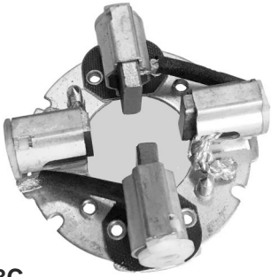
P2178C PORTAESCOBILLAS ARRANQUE TIPO ISKRA
