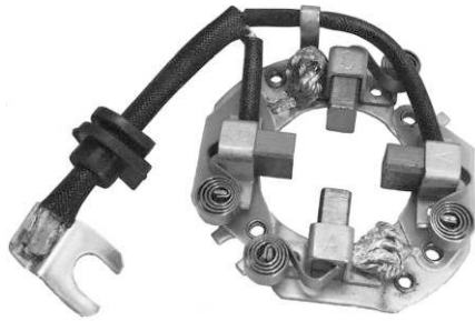
P2407C PORTAESCOBILLAS ARRANQUE TIPO HITACHI
