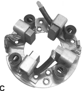
P2403C PORTAESCOBILLAS ARRANQUE TIPO NIPPONDENSO
