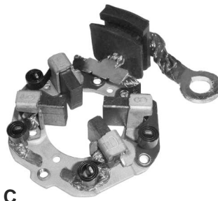
P2351C ARR. HITACHI 5,5 x 14,4 x 14,8
