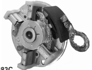
P2383C ARR. VALEO NISSAN, CLIO, LOGAN, SANDERO, ECOSPORT 2002-2012 5 x 12 x 11,6
