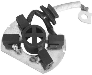
P2140C ARR. BOSCH, CHEVROLET MONTANA, FIORINO 1.3 FIRE 4,5 x 8,7 x 10,5 12v.
