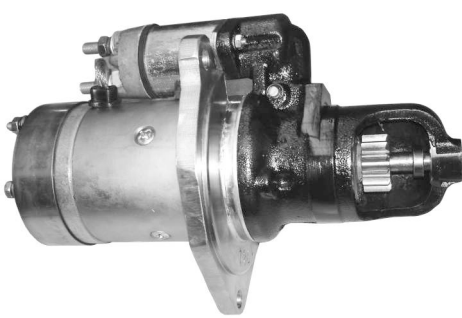
301782 FIAT 780/650 - Reemplazo M.MARELL c/suncho 24V-Z12-Ø43,5 301782/12 ÍDEM 12V
