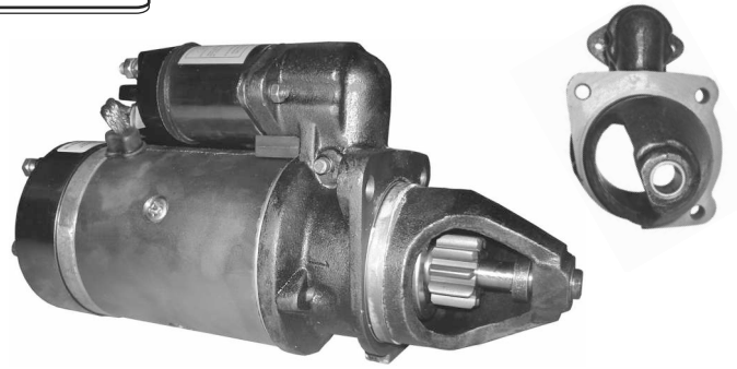
301040 BEDFORD CIMARRÓN CHEVROLET 12V-Z10-Ø40 Reforma AN115 (35256060)
