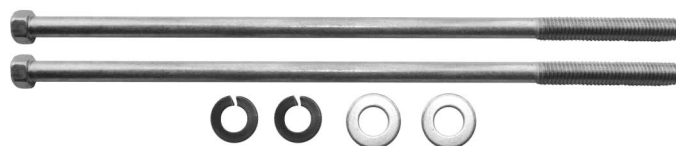
T2123 ARRANQUE TIPO BOSCH, IME, RASTROJERO MOTOR INDENOR Y BORGWARD M6X168MM. CABEZA HEXAGONAL (Cant. 2)
