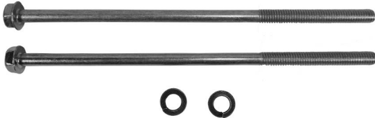
T2219 ARRANQUE TIPO INDIEL / PRESTOLITE M100R M6X145MM. (Cant. 2)
