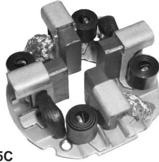
P2355C ARR. MITSUBISHI 8 x 24 x 17,5
