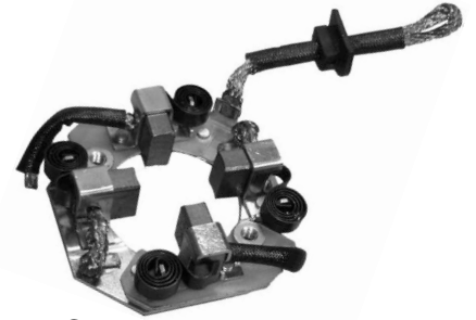
P2290C ARR. NIPPONDENSO 7 x 14 x 16.4
