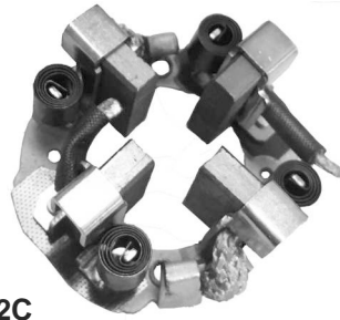
P2402C PORTAESCOBILLAS ARRANQUE TIPO NIPPONDENSO
