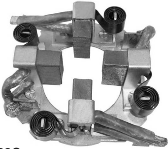
P2388C PORTAESCOBILLAS ARRANQUE TIPO ISKRA
