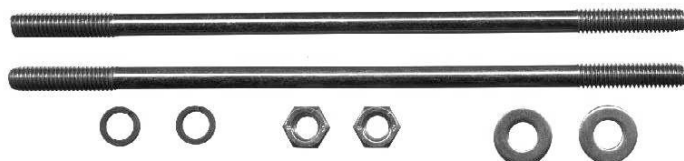
T2191 ARRANQUE TIPO GAREF FIAT 125, DOBLE ROSCA M6X158MM. (Cant. 2)
