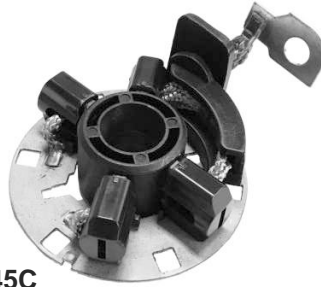
P2445C PORTAESCOBILLAS ARRANQUE TIPO BOSCH
