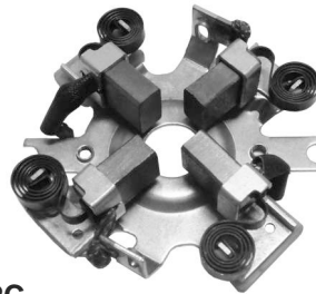
P2152C ARR. MARELLI, FIAT DUCATO, IVECO, ALLIS 9 x 16 x 23.5.
