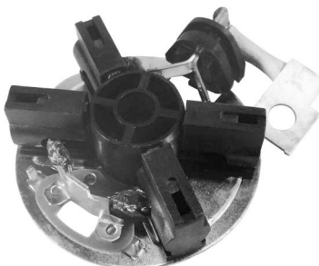
P2142C ARR. BOSCH, SCANIA (P230, 310, 340, 420) 5,5 x 28 x 18 24v.
