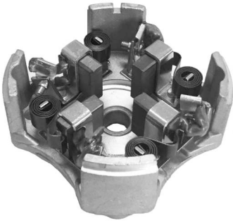
P2425C PORTAESCOBILLAS ARRANQUE TIPO BOSCH
