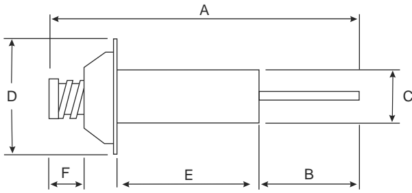
P8130 TIPO NIPPONNIPPONDENSO, ISUZU, TOYOTA, LUV, MAZDA
