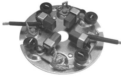
P2411C PORTAESCOBILLAS ARRANQUE TIPO BOSCH
