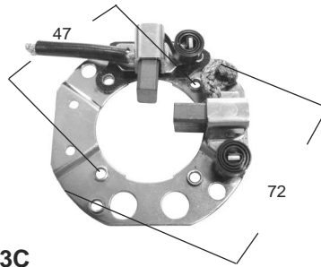
P2343C ARR. MARELLI, SIENA, PALIO 7 x 13 x 17.5 (9945553)
