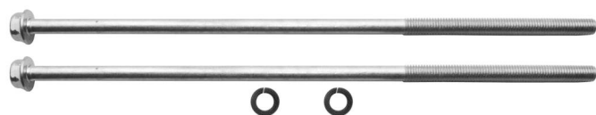
T2200 ARRANQUE TIPO INDIEL M93 FRONTAL, RENAULT 11/19 M5X166MM. (Cant. 2)
