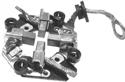
P2449C PORTAESCOBILLAS ARRANQUE TIPO EFFA
