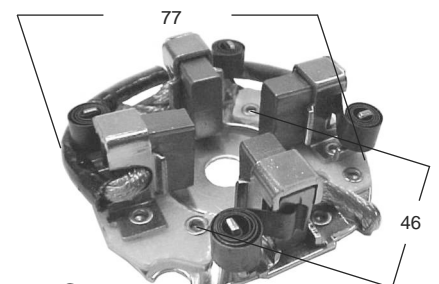
P2230C ARR. MARELLI, DUCATO, BOXER, BERLINGO 8 x 19 x 20
