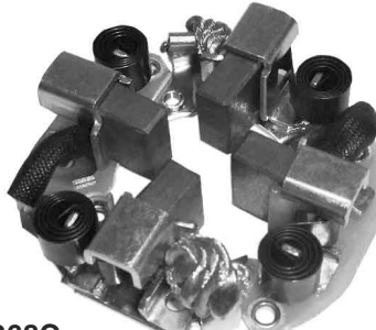
P2368C ARR. NIPPONDENSO, FIAT PALIO, CHEVROLET, ISUZU, TOYOTA. 7 x 16 x 15,5
