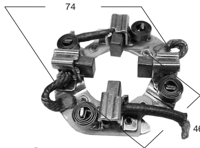
P2222C ARR. MARELLI, FIAT DUNA NAFTERO 7 x 13 x 18
