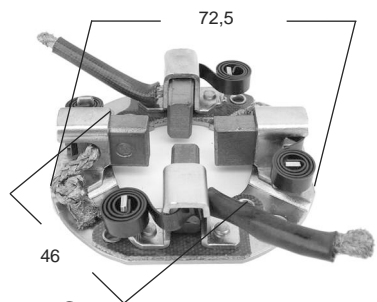
P2242C ARR. MARELLI, FIAT TIPO, PALIO SIENA 7 x 13 x 17.5 (832 212 41)
