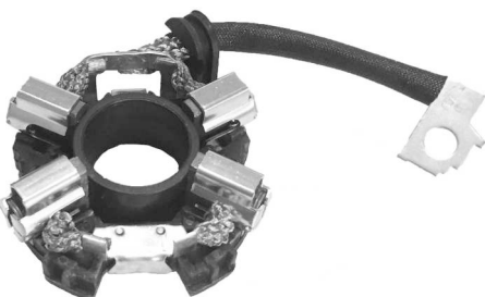
P2422C PORTAESCOBILLAS ARRANQUE TIPO BOSCH
