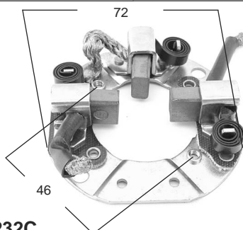
P2232C ARR. MITSUBISHI, TOYOTA 7 x 10 x 16 (3 carbones) (M649T04471)
