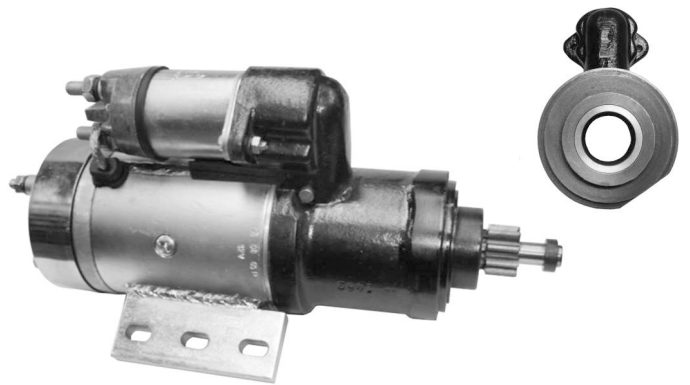
301430 DEUTZ DA130-144-514 MOTOR 1113-2114 24V-Z9-Ø34,5 (REEMPLAZO ARR. BNG. C/SUNCHO)
