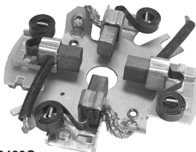
P2423C PORTAESCOBILLAS ARRANQUE TIPO BOSCH
