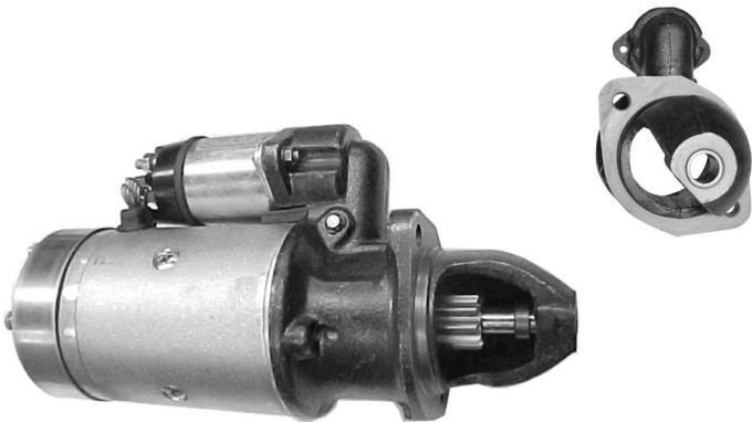
301471 FIAT U25 - GIRO IZQUIERDO 12V-Z9-Ø34,5
