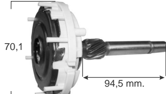
P1406 BOSCH, GOLF (F000 AL0 128 - 1 006 200 128 F 000 AL0 128)
