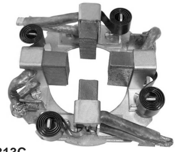
P2313C PORTAESCOBILLAS ARRANQUE TIPO ISKRA
