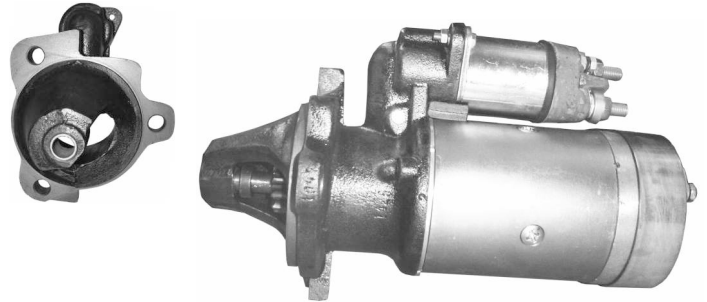
301047 FIAT 619 - Reemp. arranque FKB 24V Z11 Ø40,8 - Ref. DIPRA
