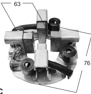
P2246C ARR. MITSUBISHI, FORD VAN 8 x 24 x 18 12v (F4TZ-11061-A SBE-351)
