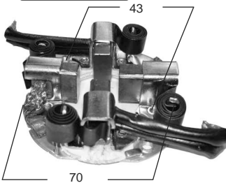
P2134C ARR. VALEO, RENAULT TRAFIC DIESEL, TRIO, EXPRESS. 9 x 22 x 18 (1 004 336 801 / 821 / 827 / 951 F 000 AL 1 051)
