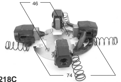
P2218C ARR. INDIEL M93R, MOTOR MAXION (casillero baquelita) 8 x 19 x 18 (352 58 637)
