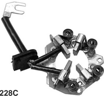
P2228C PORTAESCOBILLAS ARRANQUE TIPO NIPPONDENSO
