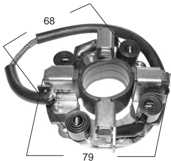
P2395C ARR. INDIEL 7.8 x 24.8 x 21 (K-01260)
