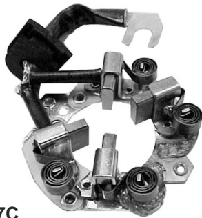
P2137C PORTAESCOBILLAS ARRANQUE TIPO HITACHI - INDIEL
