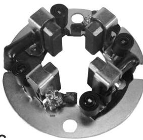
P2311C ARR. NIPPONDENSO, KIA, DAIHATSU 8 x 25 x 15.5 12v.
