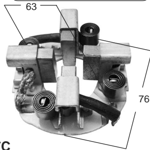
P2247C ARR. MITSUBISHI, FORD VAN 8 x 24 x 18 24v.
