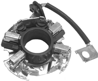
P2416C PORTAESCOBILLAS ARRANQUE TIPO BOSCH
