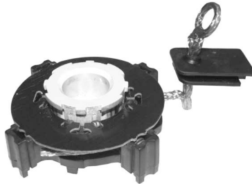
P2345C ARR. VALEO, ESCORT, FIESTA, KA 6.5 x 8 x 11 (3 carbones, colilla 40 mm) (594290)
