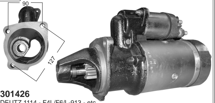
301426/12 ÍDEM 12V (35256747) 301426B/12 ÍDEM BLINDADO 12V
