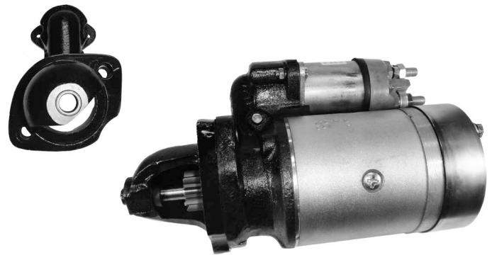
301472 FIAT 411-24V-Z9-Ø35
