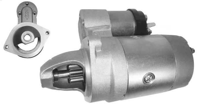
300160/5 PEUGEOT 504 - 505 FRONTAL - 12V-Z9-Ø25,5
