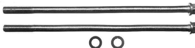
T2203 ARRANQUE TIPO BOSCH INDIEL, HITACHI M74 VARIOS M5X125MM. CABEZA HEXAGONAL (Cant. 2)
