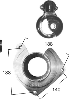
301783 FIAT 780 Reemplazo BPD 24V-Z11-Ø40,8
