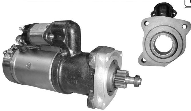
301469I FIAT 650-700 / Reemp. CAV GIRO IZQ. 12V-Z10-Ø38,5 - Ref. AN115
