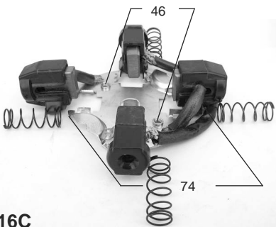
P2216C ARR. MARELLI, FIAT DUCATO 8 x 19 x 18 (855 403 41) (casillero baquelita)
