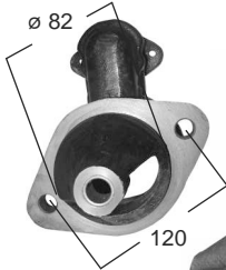
301068 J.DEERE 1420-2030-2144-2333-2420-2530-2730-3140 12V-Z10-Ø32
