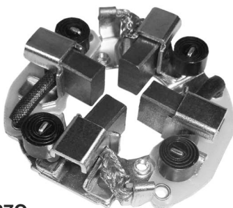
P2367C ARR. NIPPONDENSO ISUZU, TOYOTA, SUZUKI, KUBOTA. 7 x 13 x 15,5
