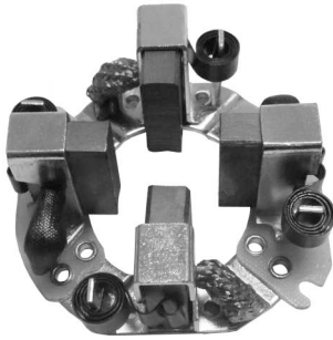
P2159C ARR. HITACHI 10 x 35 x 22
