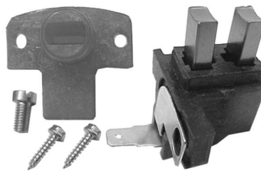
P7116 ALTERNADOR GAREF FIAT - PEUGEOT - COMPLETO
