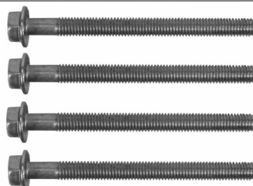
T5205 ALTERNADOR TIPO BOSCH M5X60MM. CABEZA HEXAGONAL (CANT.4)
