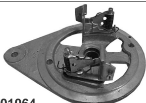
701064 TAPA PORTA CARBON DE DINAMO CHEVROLET, IKA, ESTANCIERA
