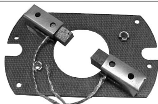
MAB1009 PORTAESCOBILLAS ALTA Y BAJA CANADIENSE
