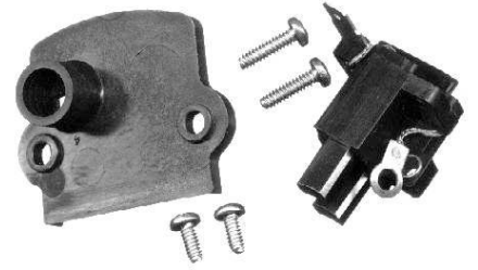
P7004 ALT. INDIEL 28/55/70 amp. FORD FALCON - F100 - PERKINS - PEUG.- FIAT - COMPLETO
