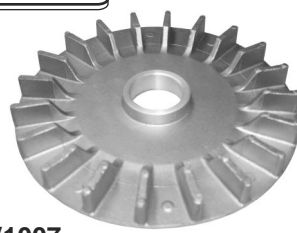
V1007 TIPO BOSCH, WAPSA 24V. 75A. M. BENZ EJE 30MM.
