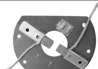
MAB1001 PORTAESCOBILLAS ALTA Y BAJA TIPO ROHER
