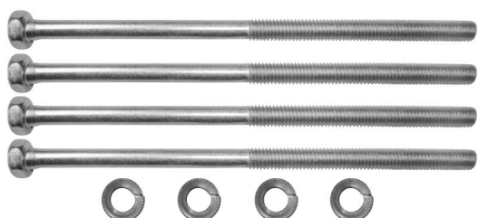
T5221 ALTERNADOR TIPO BOSCH VARIOS 24V. 90A. M6X125MM. CABEZA HEXAGONAL (CANT. 4)
