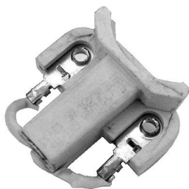
P7146 FORD - F250 / F350 / RANGER (F1D2-10347- A-GB 320) IR/IF 36 SERIE - 4x7.5x18 F1DZ-10347-A
