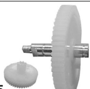
LP1055 JUEGO BUFFALO (TODOS). ENGRANAJE GDE.: Z64, Ø50MM. ENGRANAJE MED.: Z47 Ø28.3MM. ENGRANAJE CHICO: Z7 Ø7MM. EJE: LARGO 23.5MM. Ø8MM.
