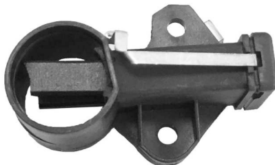
P7171 PORTAESCOBILLAS ALTERNADOR TIPO DELCO REMY
