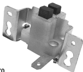
P7170 ALT. VALEO, MOTOROLA 8AL/P 8AR 5,3 X 6,8 X 15
