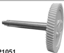
LP1051 CHEVROLET 400, CHEVY - BRIEVA. ENGRANAJE: Z70 Ø66MM. EJE: LARGO 91.3. Ø11.3MM.
