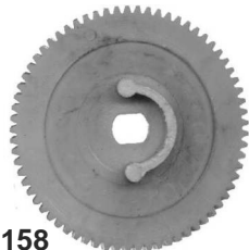
LP1158 DODGE CAMION, POLARA. ENGRANAJE: Z69 Ø82.6MM.
