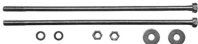
T8195 TORNILLOS PASANTES DINAMO FIAT 600 M5X163MM. (CANT. 2)
