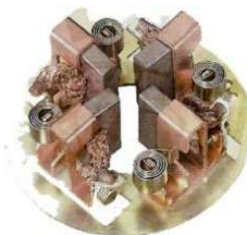
12336 - BOSCH
